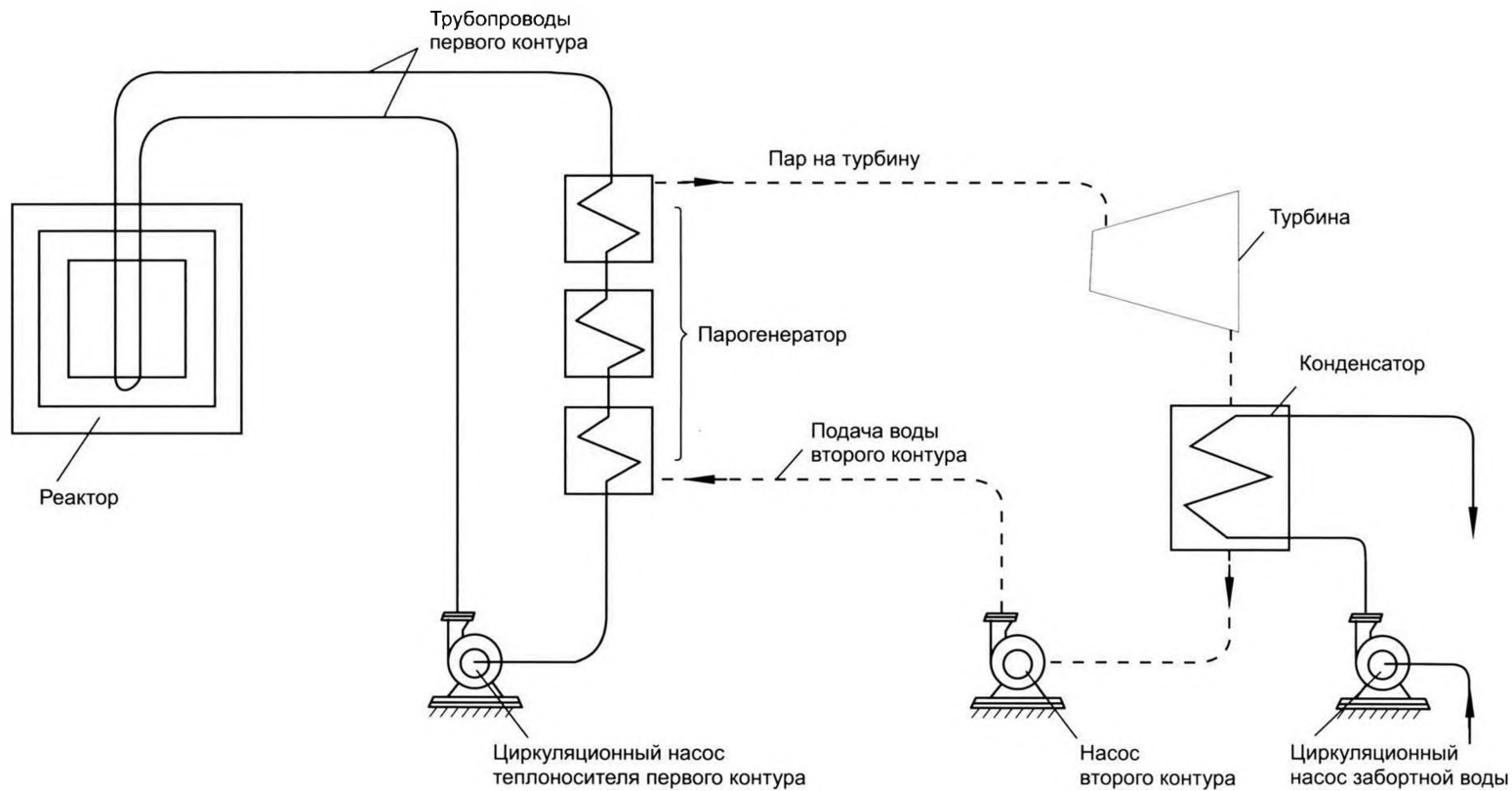
Рис. 1. Принципиальная схема ЯЭУ (предсказный проект)
