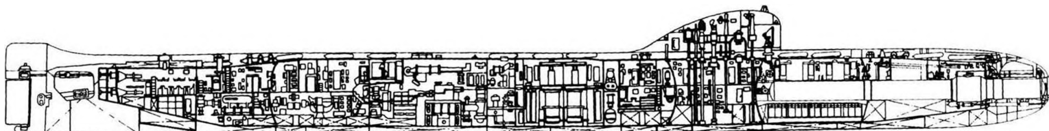
Рис. 9. АПЛ пр. 627. Общее расположение. Продольный разрез (технический проект до корректировки)
