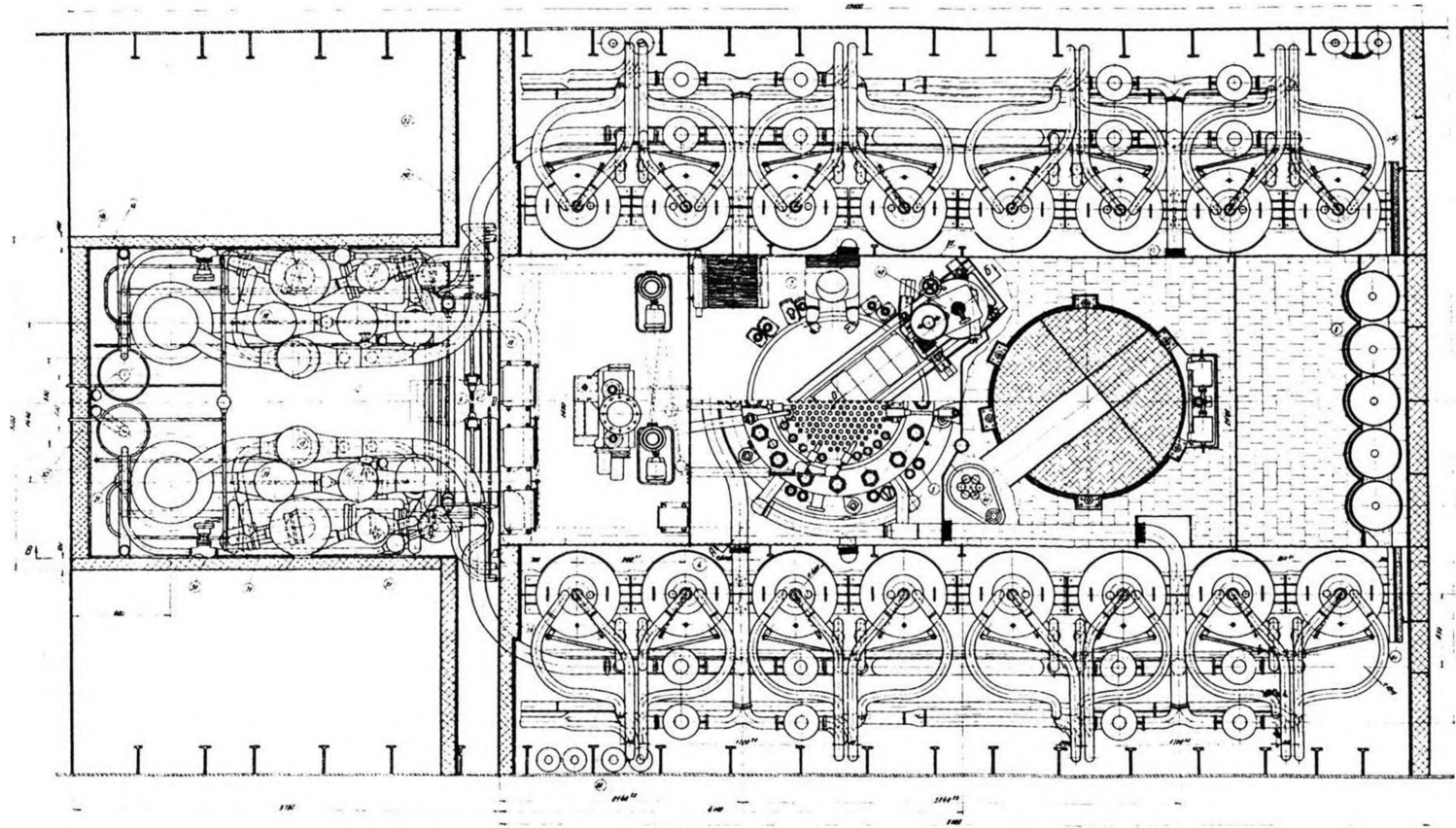
Рис. 5. Компоновка ППУ в отсеке. План (технический проект)
