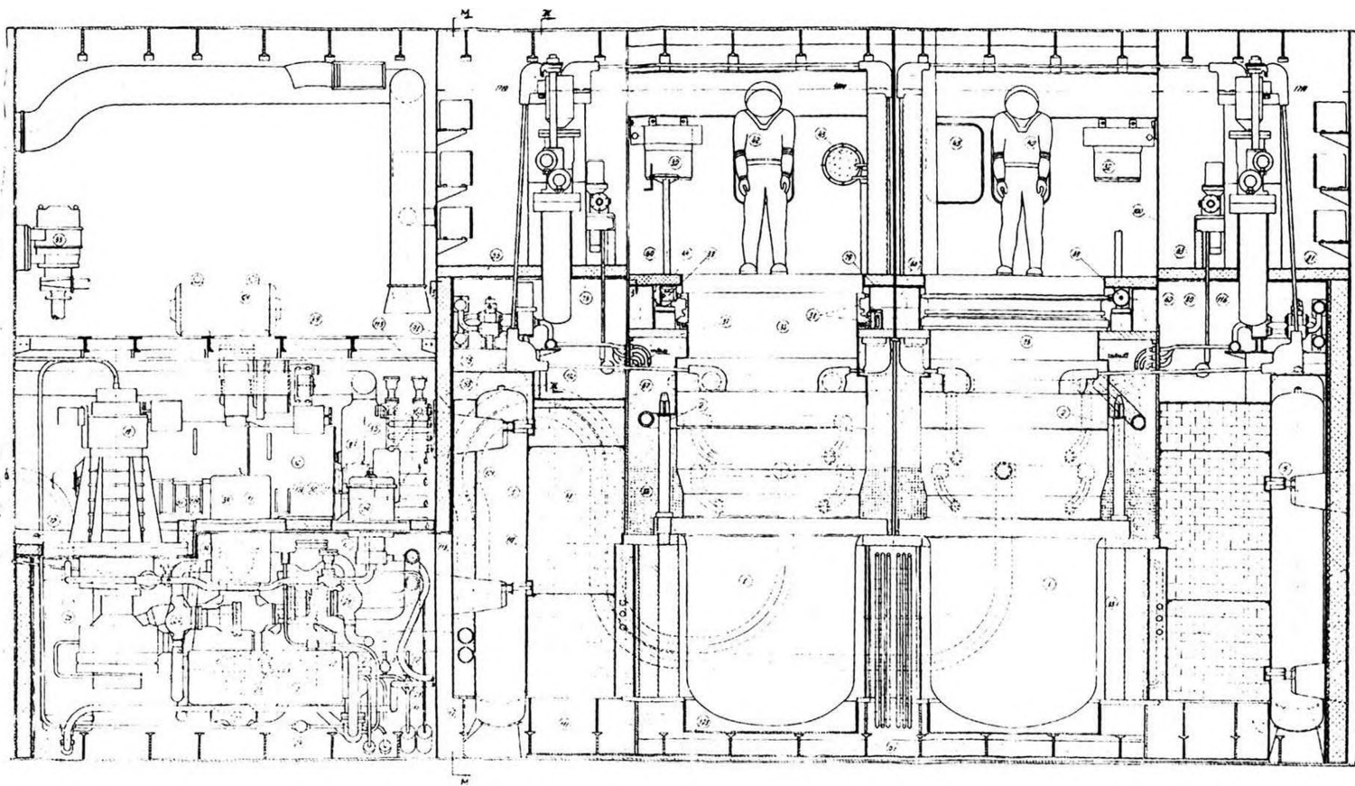
Рис. 4. Компоновка ППУ в отсеке. Продольный разрез (технический проект)
