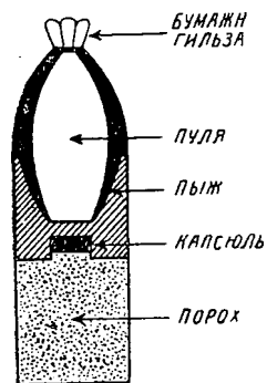
Черт. 13. Патрон к ружью Дрейзе.
