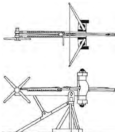
Полибол (полуавтоматический стреломёт)
