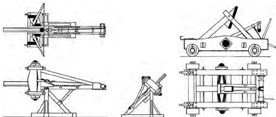
Корабельный одноплечевой торсионный камнеёт-онагр
