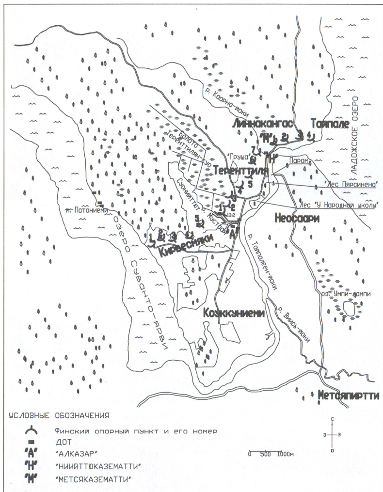
Схема финских оборонительных позиций в районе Тайпале. Фото автора
