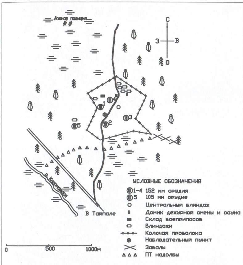
План территории батареи «Каарнайоки». Из архива автора
