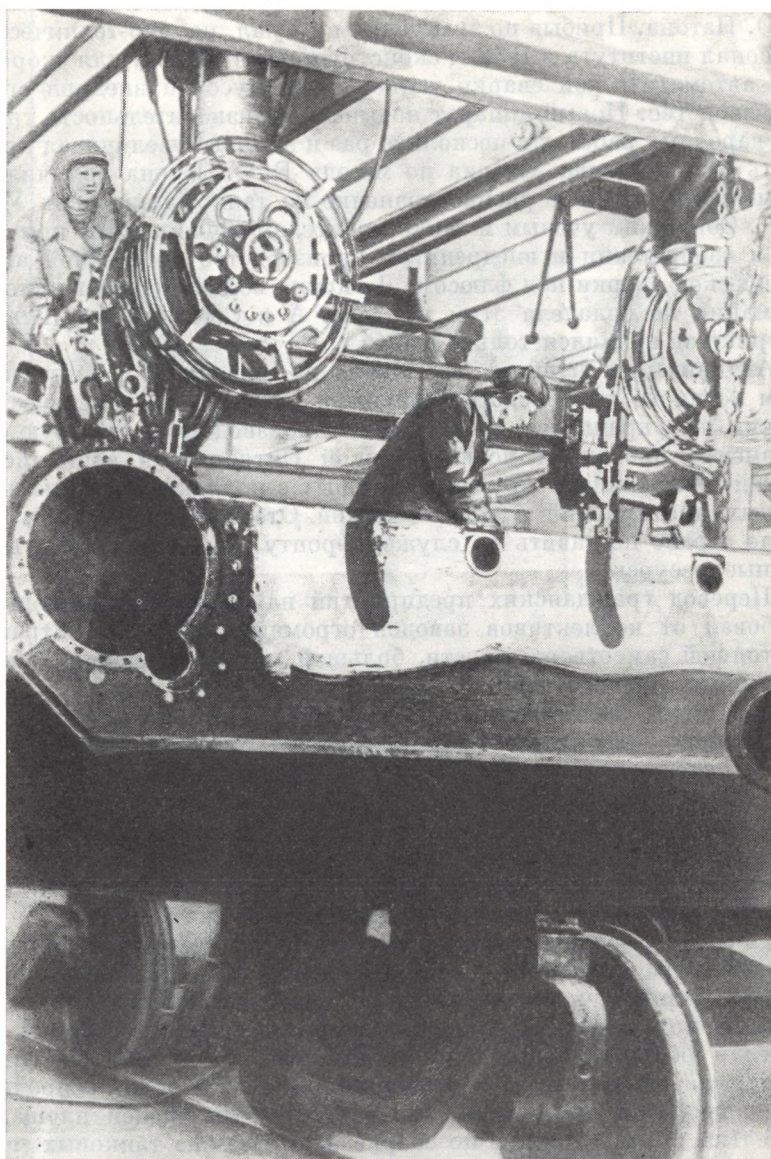
Обработка корпуса танка Т-34 с помощью аппарата автоматической сварки академика Е. О. Патона
