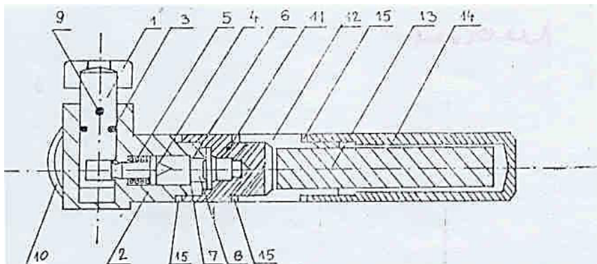
Илика 146. — Upaljač specijalni hemijski nagazni — 1 (USHN — 1): 1 — klip, 2 — smjesa, 3 — pokrivka, 4 — udarna igla, 5 — opruga, 6 — nosač smješe, 7 — pokrivka, 8 — nosač smješe, 9 — osigurač, 10 — alka, 11 — šep osigurača, 12 — nosač detonatorske kapsle, 13 — detonatorska kapsla, 14 — zaštitna kapa, 15 — zaptivač
