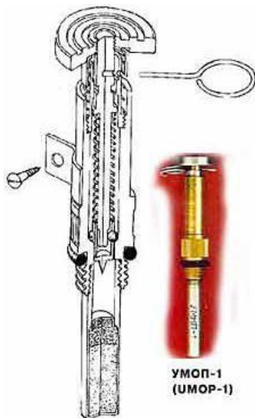
ФОТО 127. Взрыватель УМОП-1 / Ю.Г.Веремеев
