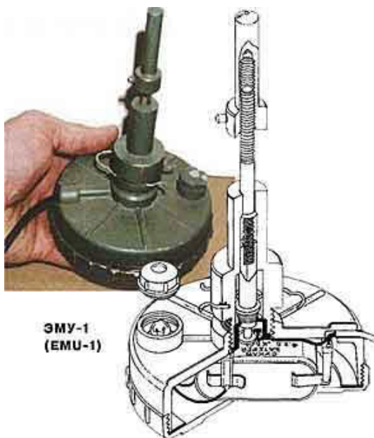
ФОТО 136. Электромеханический взрыватель ЭМУ-1 / Ю.Г. Веремеев
