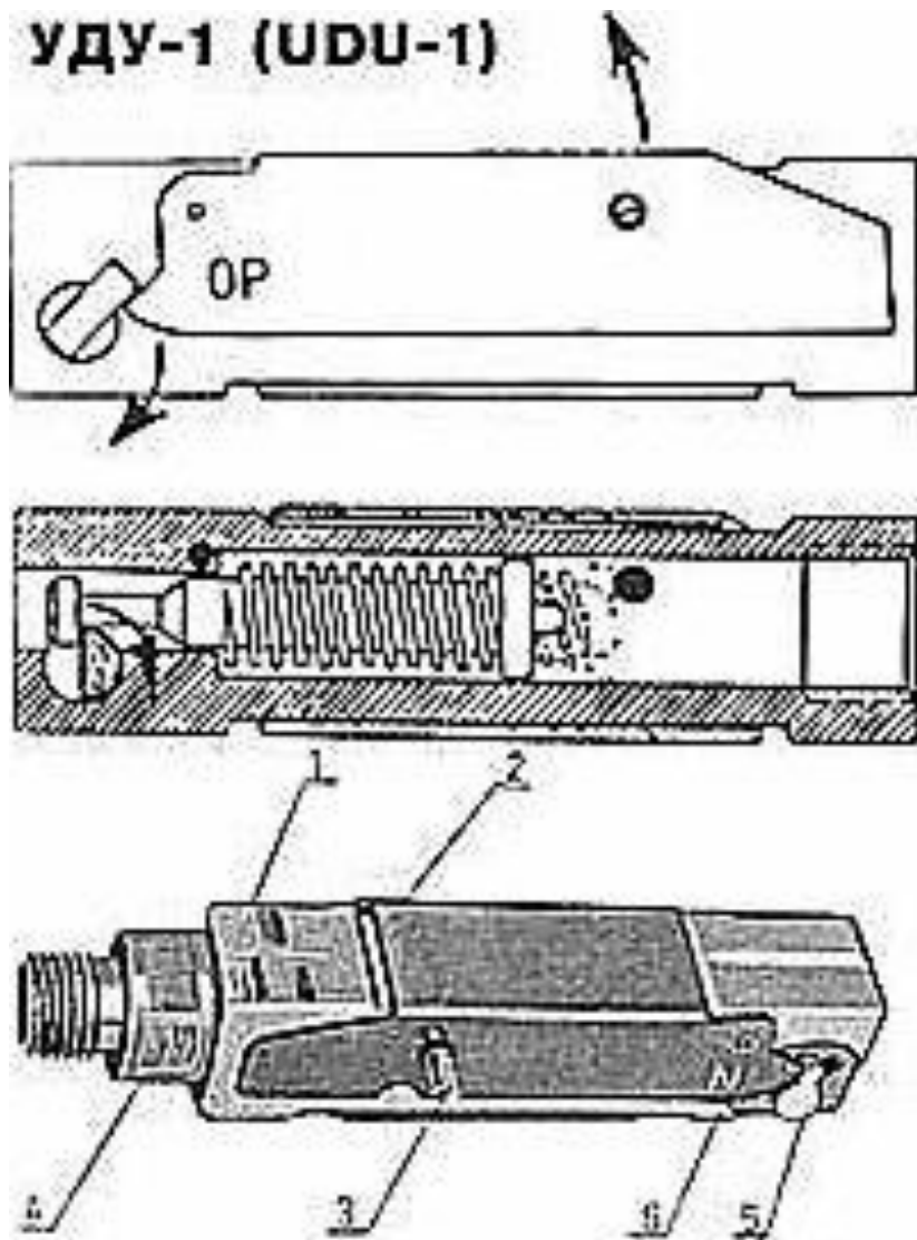
ФОТО 124. Взрыватель УДУ-1
