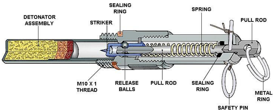
ФОТО 128. Взрыватель УМП-1
