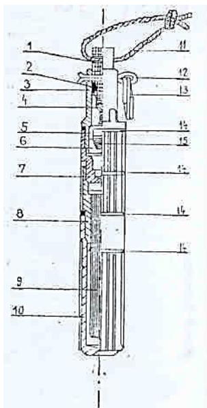
Slika 145. — Upaljač specijalni hemijski potezni — (USHP-1): 1 — potezač, 2 — telo upaljača, 3 — zaptivač, 4 — potezna žica, 5 — nosač smeše, 6 — zapaljiva smeša, 7 — čep osigurača, 8 — nosač detonatorske kapsle, 9 — detonatorska kapsla, 10 — zaštitna kapa, 11 — kanap za potezanje, 12 — osigurač, 13 — alka, 14 — zaptivač
