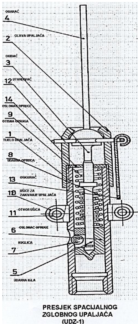
ФОТО 132. Взрыватель штыревой УДЗ-1 // Stevanović Trajko, Petrović Svetislav. Priručnik minskoekspozivnih sredstava / Zavod za udžbena i nastavna sredstva. Beograd, 1987
