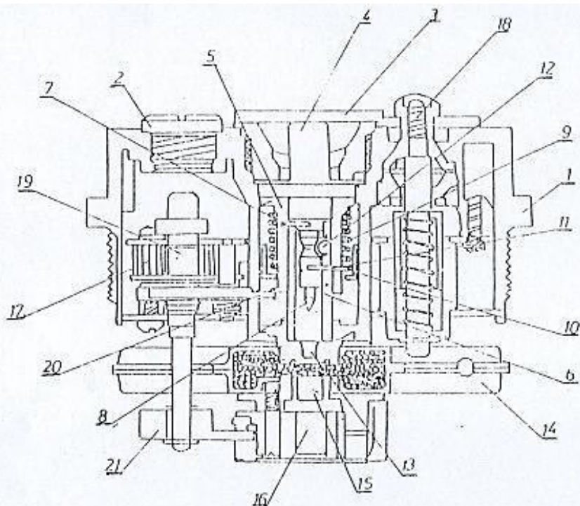
Слика 109. — Упалјач противтенковске разорно-пробожне мине — 6 (УТМРП — 6): 1 — тело, 2 — заштитни њеп, 3 — заштитна капа, 4 — носач полуге, 5 — клизач, 6 — водича, 7 — џивија клизача, 8 — ударна игла, 9 — ударна опруга, 10 — пластично џауње, 11 — џивија ударне игле, 12 — осигуравајућа куглица, 13 — иницијална капсула, 14 — избачно пулjenje, 15 — успораџ, 16 — детонаторска капсула, 17 — сатни ме- ханизам, 18 — starter, 19 — главна осовина, 20 — сигурносна полуга, 21 — полу- кружни брег
