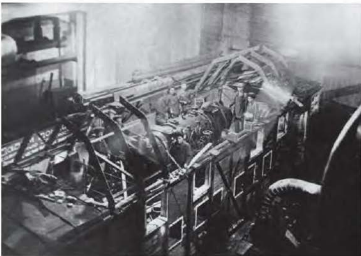
Сборка энергопоезда для Донбасса, декабрь 1943 г.
