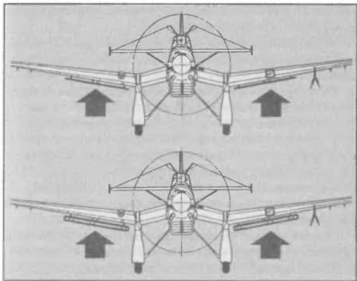
Воздушные тормоза на крыльях Ю-87. Вверху – убраны, внизу – выпущены
