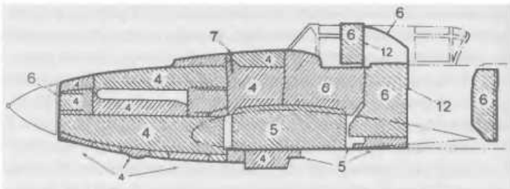
Толщина панелей бронекорпуса двухместного Ил-2 (в мм)
