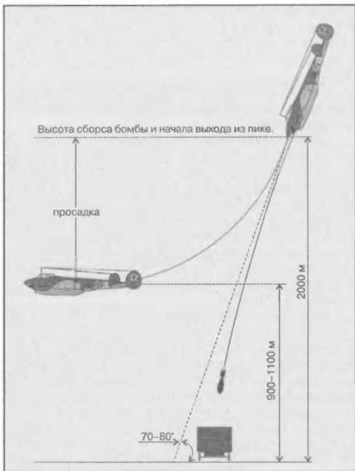
Просадка самолета при выходе из пике
