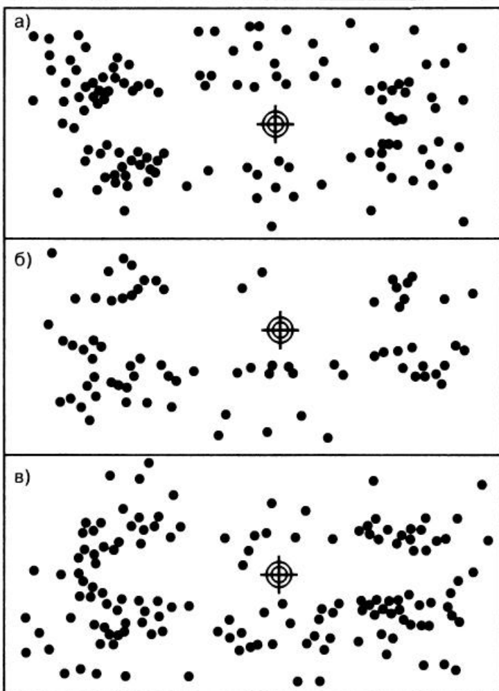
Схема отклонений авиабомб от точки прицеливания на линкоре «Октябрьская революция» во время авиационных налетов 21.09.41 г. (а), 22.09.41 г. (б) и 23.09.41 г. (в)
