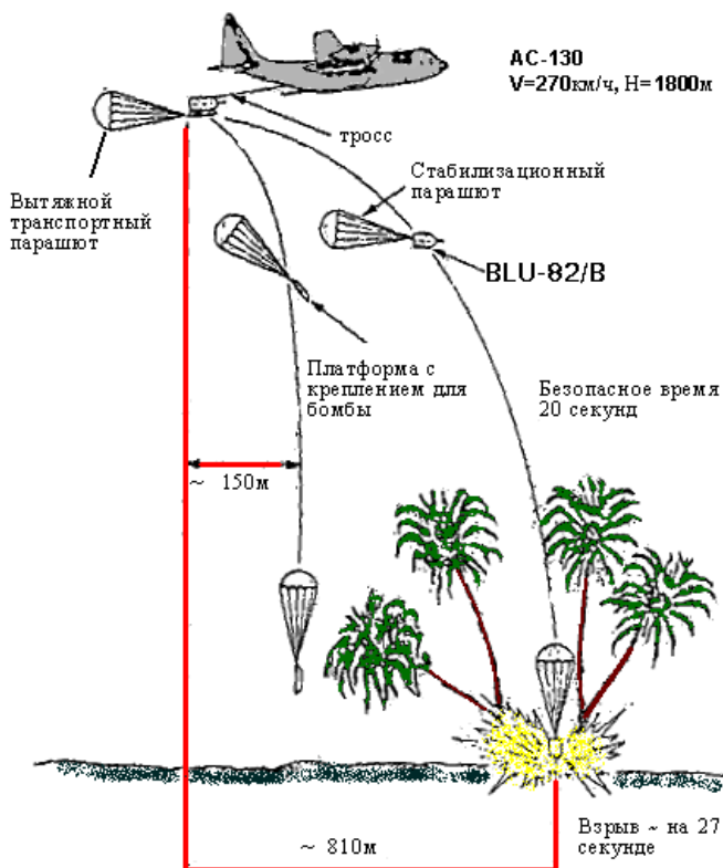
РИСУНКО 3.4. Схема сброса бомбы BLU-82 Daisy Cutter
