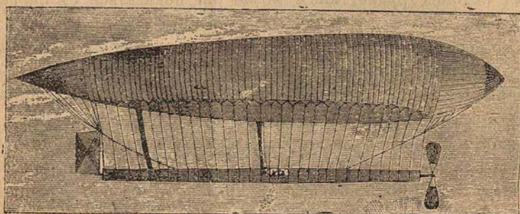
Аэростатъ Ренара и Кребса „France“.
