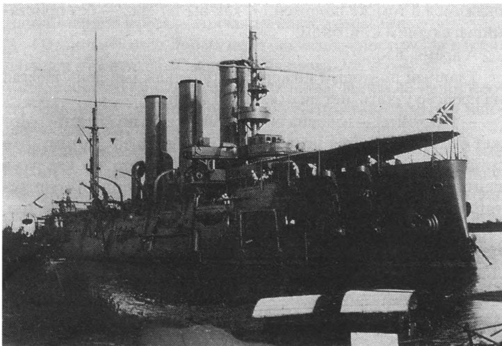
Бронепалубный крейсер 1-го ранга «Диана» (однотипный с бронепалубным крейсером 1-го ранга «Аврора») после интернирования в Сайгоне после боя в Желтом море 28 июля (10 августа) 1904 года.
