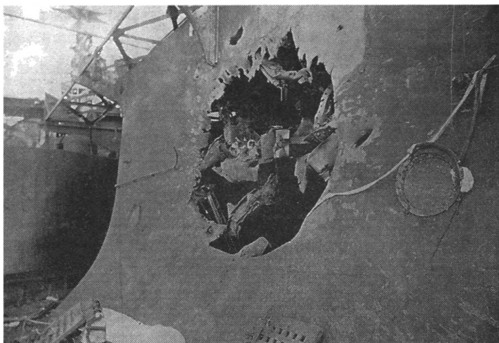
Повреждения эскадренного броненосца «Орел» в Цусимском сражении
