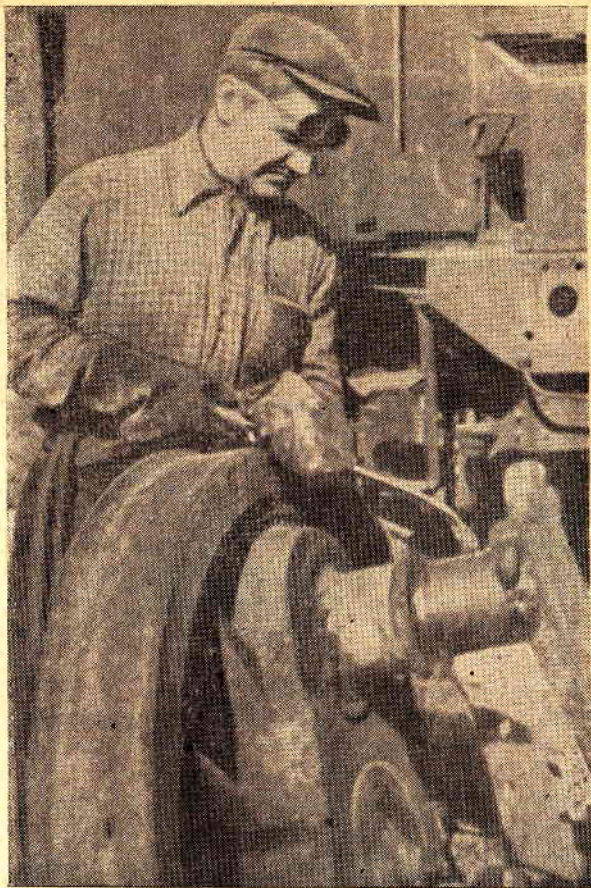
Газосварщик паровозного депо В. М. Косарев.
