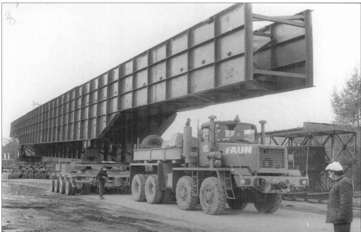
Доставка к месту монтажа балки «Мамонт» длиной 70 м, высотой 4 м и весом вместе с траверсой 180 т. Октябрь 1986 г.
