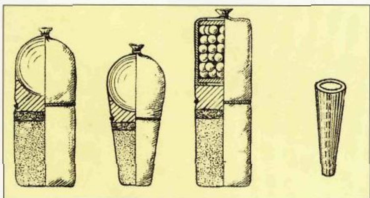
Выстрелы унитарного заряжания
