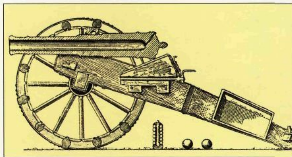
12-фунтовая пушка малой пропорции в разрезе
