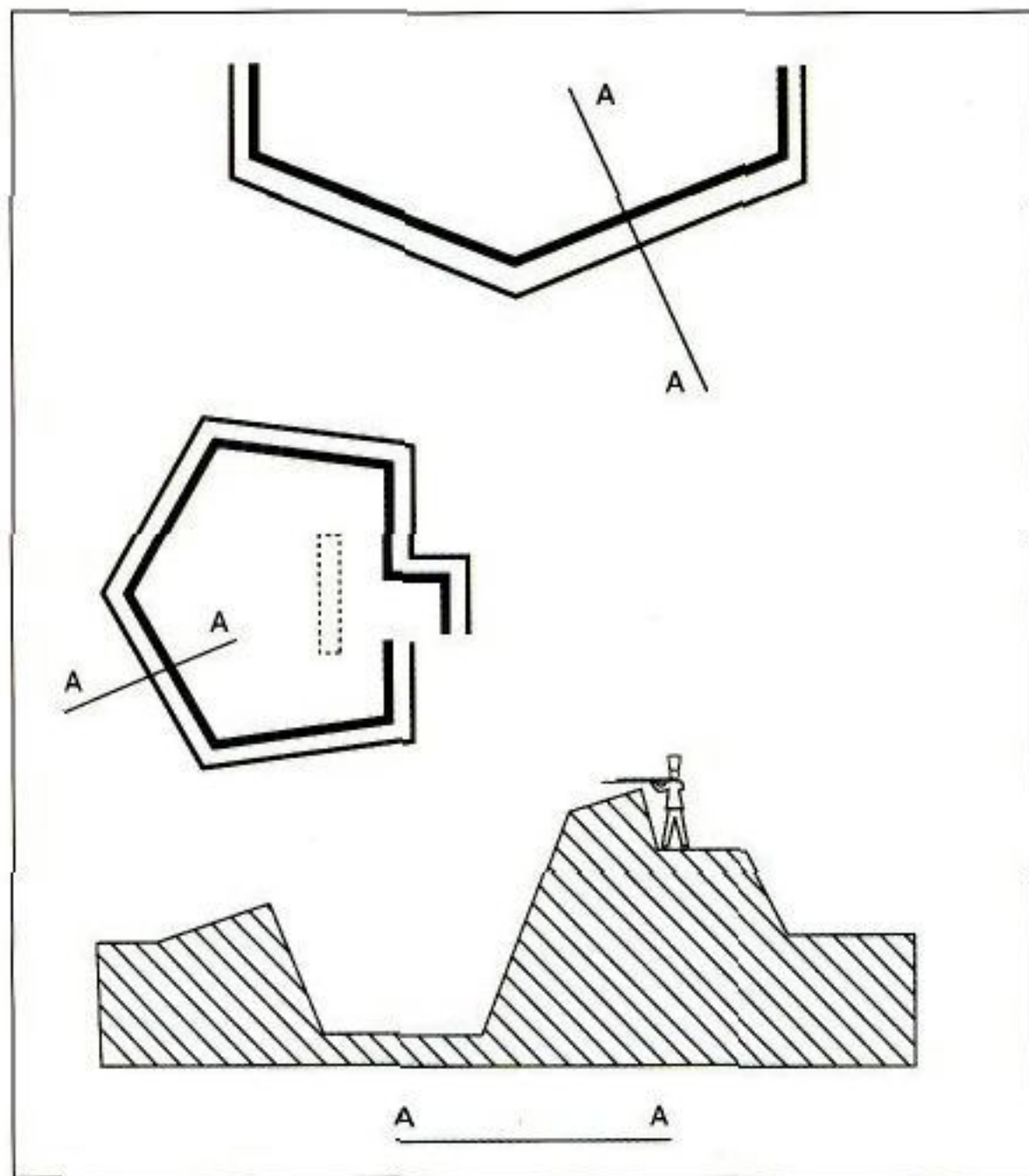
Редут и люнет
