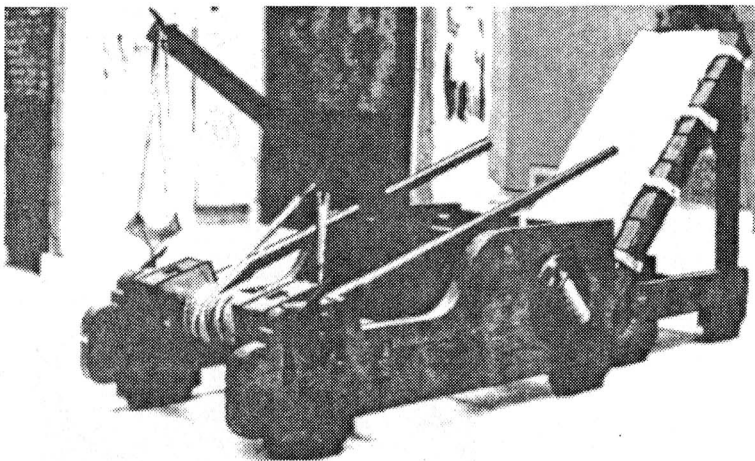
Модель римского метательного орудия (онагр).
