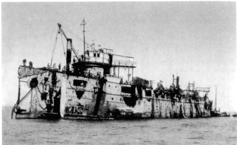
Крейсер «Варяг», поднятый со дна. 1905 г.
