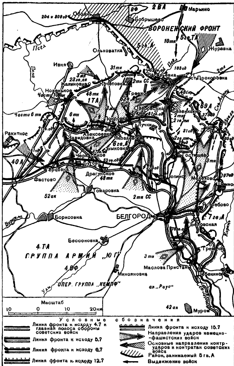
Схема 3. Оборонительное сражение на белгородско-курском направлении (5—23 июля 1943 г.)
