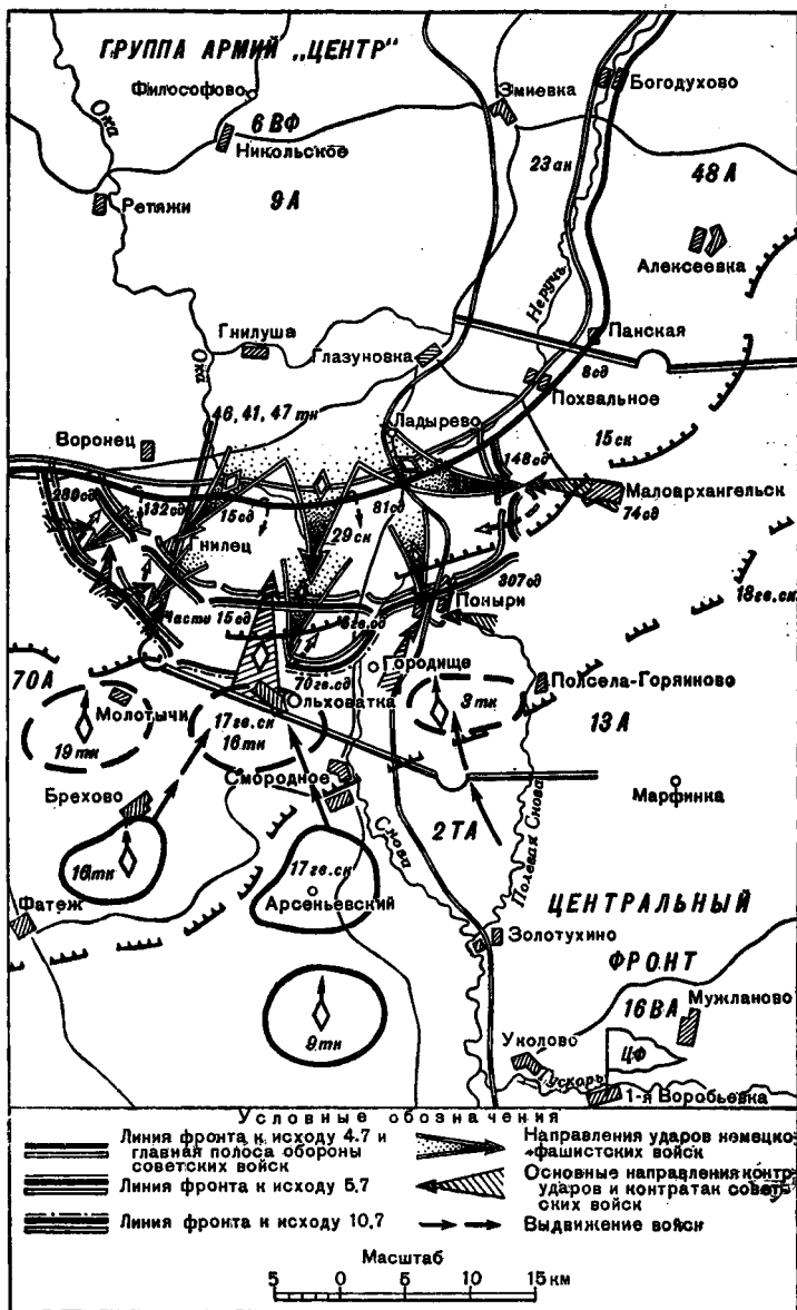
Схема 2. Оборонительное сражение на орловско-курском направлении (5—15 июля 1943 г.)
