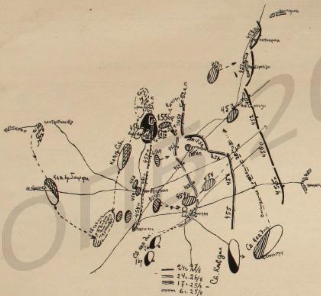
Расположение частей группы Блюхера с 25—28 августа (наступательный марш)
