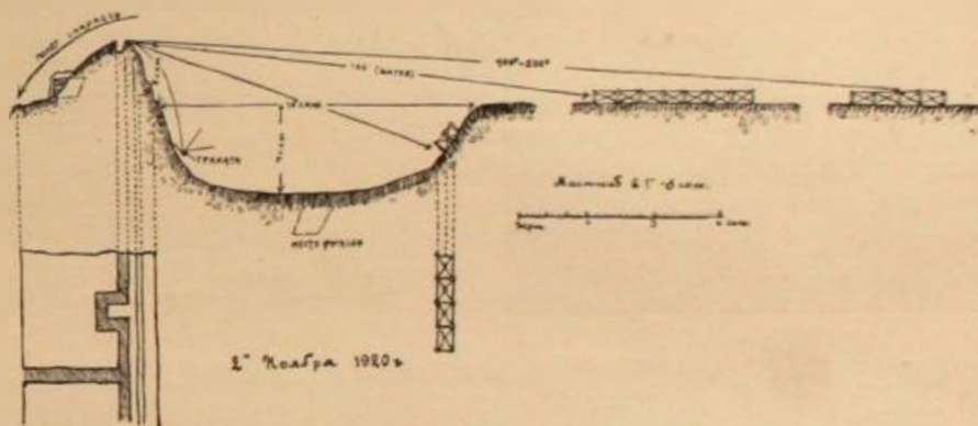
СХЕМА ПРОФИЛЯ ПЕРЕКОПСКОГО ВАЛА
