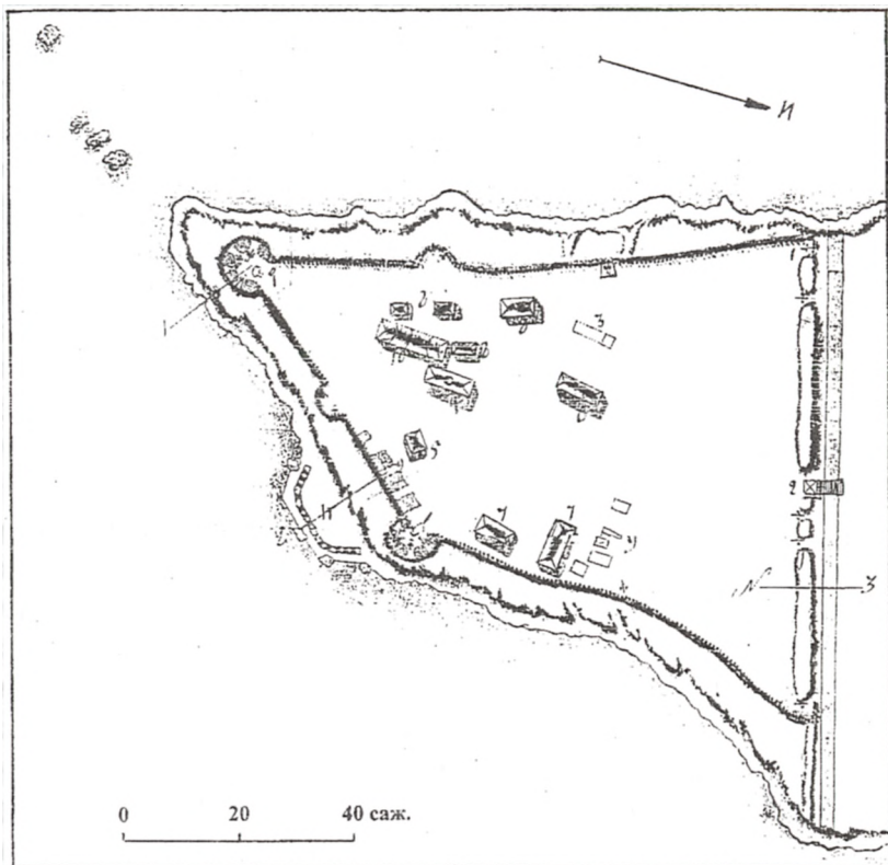
Рис. 8.. Общий план Березанской крепости 1788 г.
