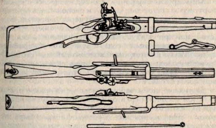
Нарезной гусарский карабин образца 1787 года. Обратите внимание на то, насколько он короче кирасирского и драгунского.
