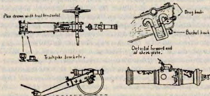
Русский четвертьпудовый «единорог» с детальным изображением гнезд для правил, крюков для накапывания и для подвешивания бабды
