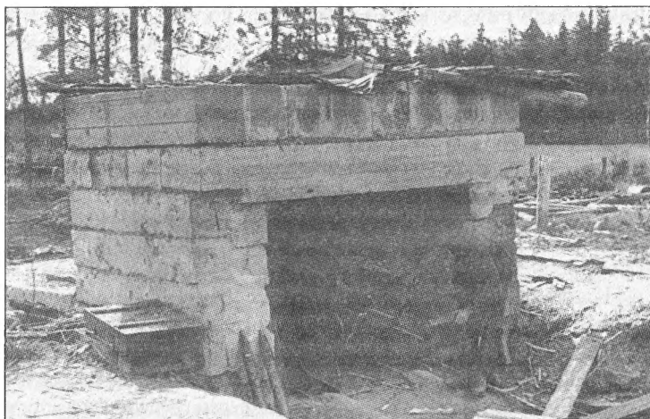
Сборная бетонная огневая точка для казематной пушки Л-17. Такие сооружения часто применялись под Ленинградом
