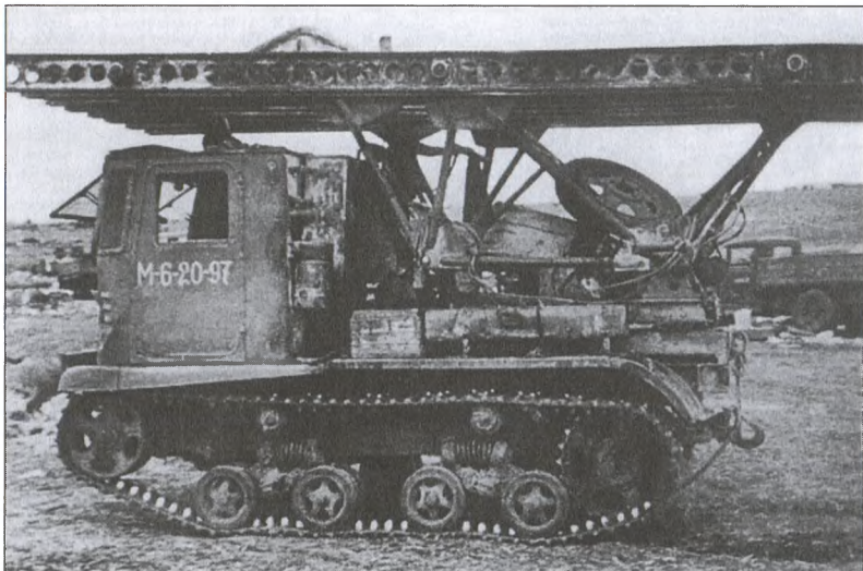
Оставленная при отступлении установка БМ-13 на базе гусеничного скоростного тягача СТЗ-5 НАТИ из состава 5-го гвардейского полка реактивной артиллерии. Номер машины: «М-6-20-97». Юго-Западное направление, конец мая 1942 года
