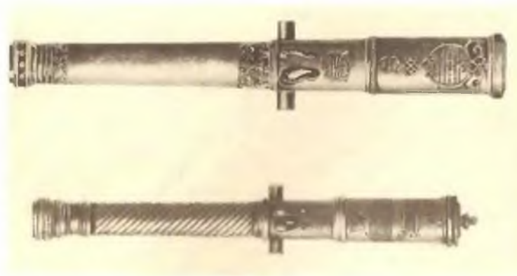
Пищаль «Гро́нд», отлитая мастером Яковом Дубиной в 1685 г. Вес 402 пуда. Старинная автография.
