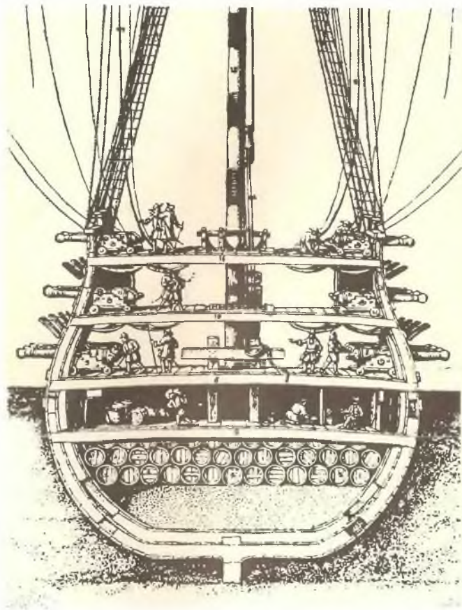
Большой парусный корабль в разрезе, XVII в. Старинный рисунок.
