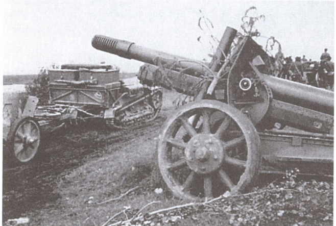
Русская 120-мм гаубица (на моторной тяге)
