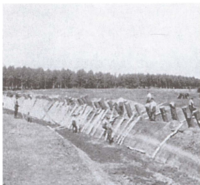
Советы ожидали нападения: противотанковые заграждения и долговременные огневые сооружения
