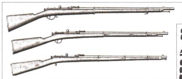
▲ Винтовки системы Бердана образца 1870 г. Сверху вниз – пехотная, драгунская, казачья.
