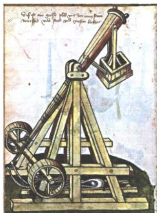
▲ Требушет. Рисунок Х. Талхоффера. 1459 г.
