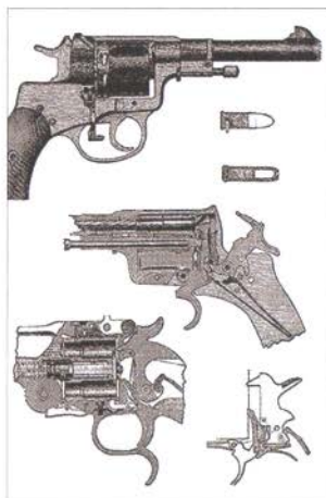
▲ Вверху и в центре – механизм револьвера системы Нагана образца 1895 г. Внизу – механизм револьвера системы Смита-Вессона образца 1869 г.
