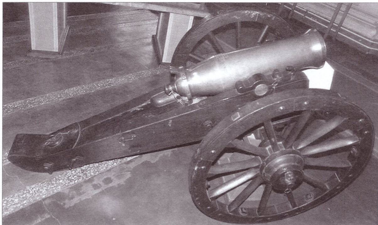
3-фунтовый (горный) единорог. ВИМАИВиВС
