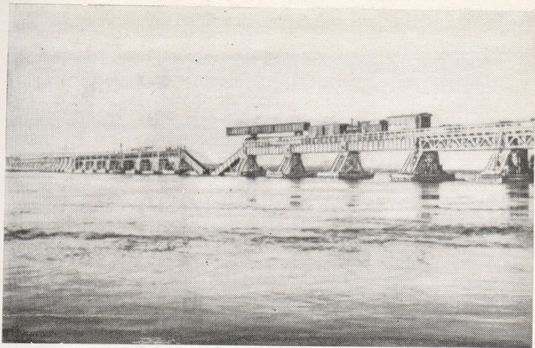
Восстановление высоковольтного моста через р. Неву, разрушенного фашистской артиллерией 25 марта 1943 г.
