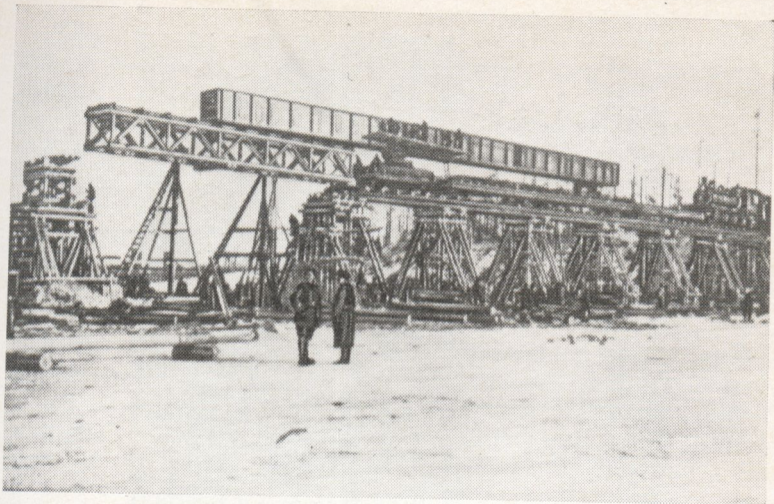
Строительство высоковольтного моста через р. Неву у Шлиссельбурга. Установка пролетного строения консольным краном.
