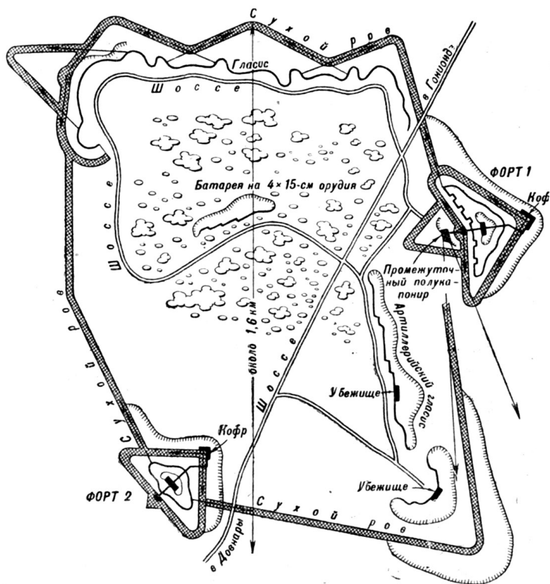
Схема 5. Опорный пункт (фесте) Гониондз
