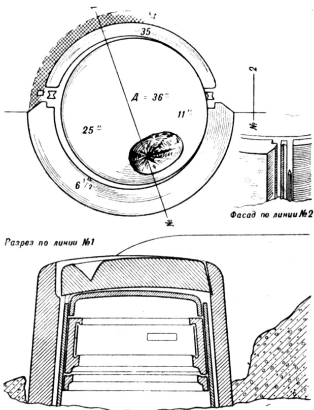
Черт. 18. Попадание 37,5-см бомбы в броневой колпак
