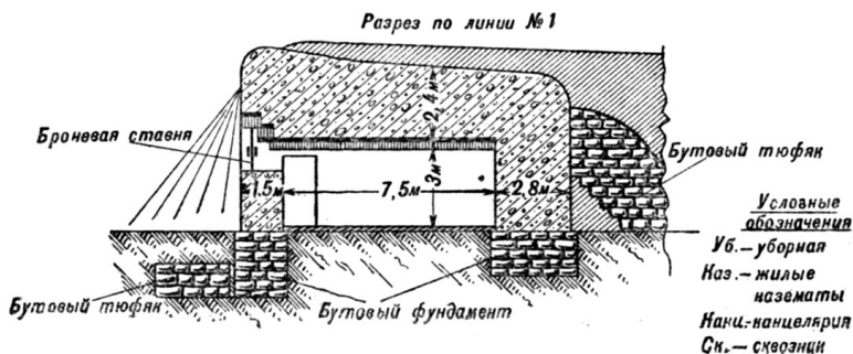
Черт. 9. Убежище на „Дровяном шоссе“
