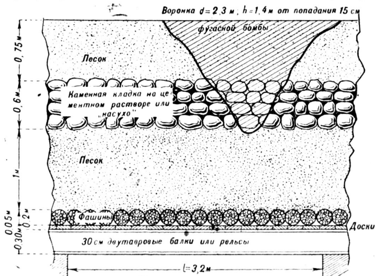
Черт. 19. Тип покрытия убежищ на Скобелевой горе
