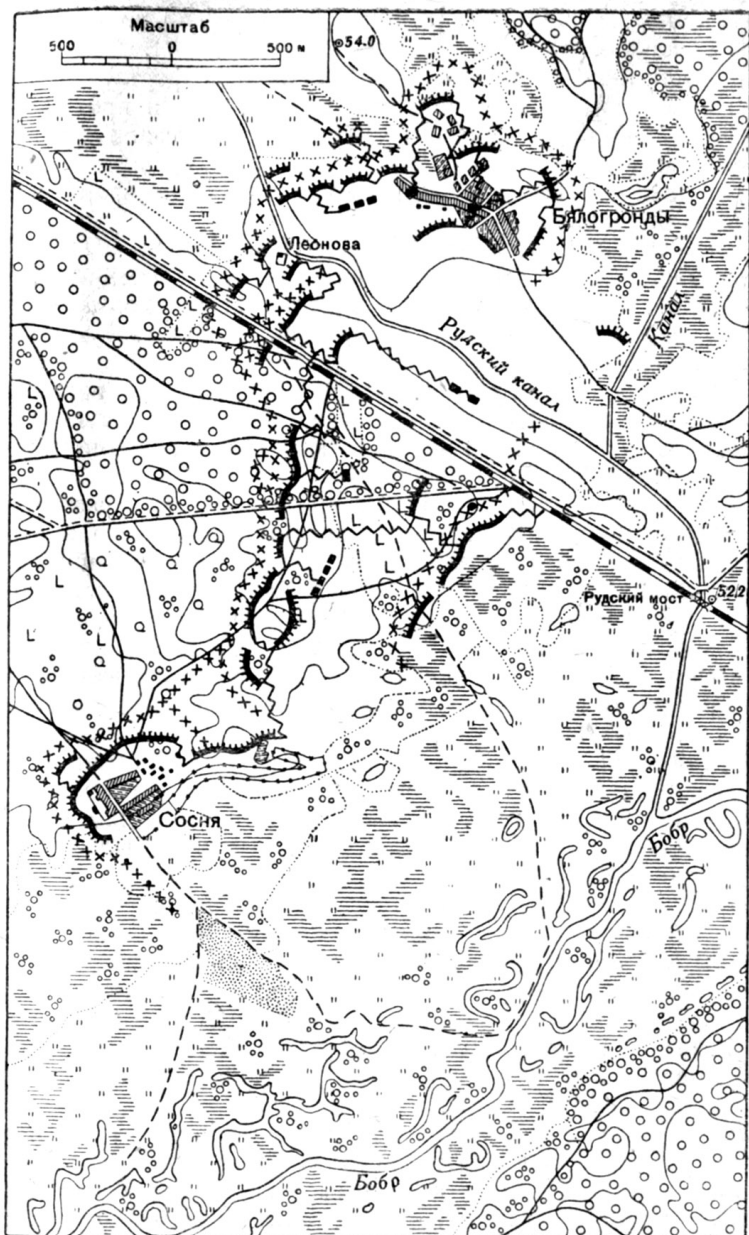
Схема 8а. Схема Сосненской позиции (левая часть)
