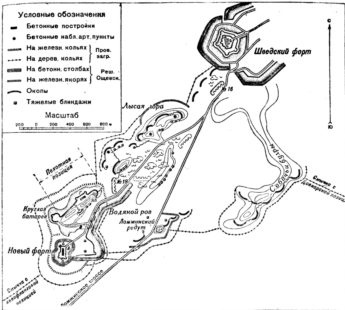
Схема 7. Схема 3-го отдела обороны
