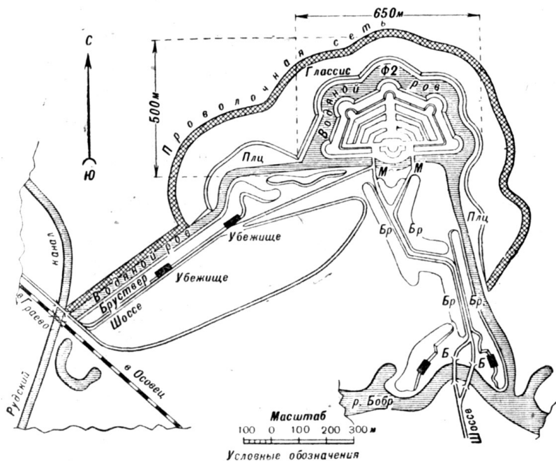
Черт. 7а. Заречный (№ 2) форт и Заречная позиция
