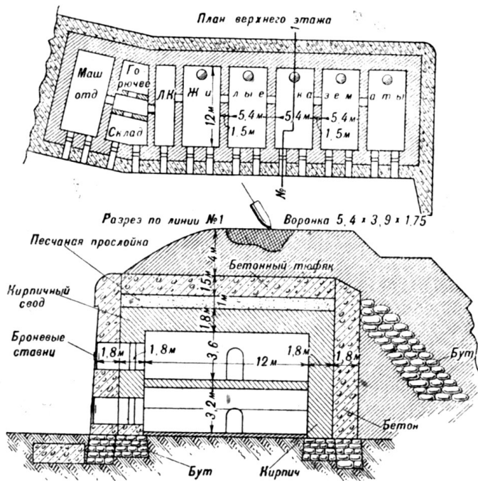
Черт. 10. Казарма № 46 Центрального форта
