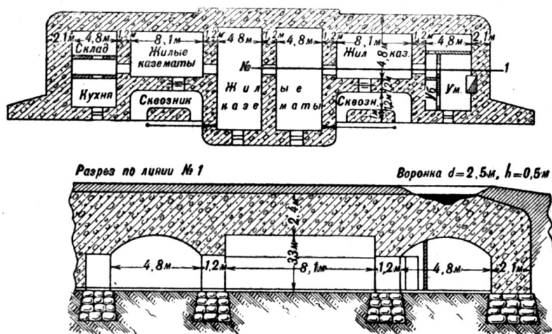
Черт. 13. Тип бетонного убежища на плацдарме
