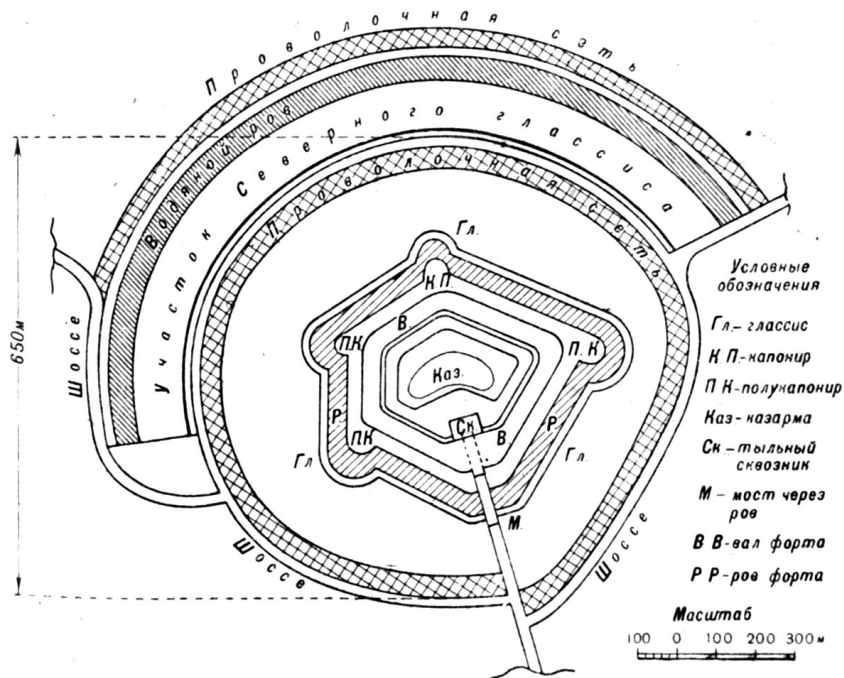
Черт. 3. Схема Шведского (№ 3) форта
