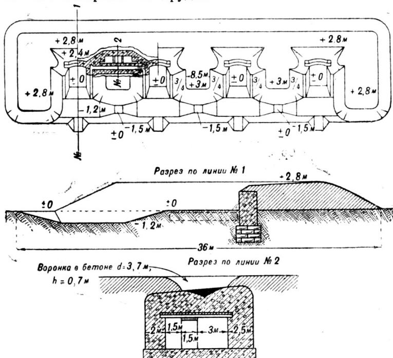
Черт. 12. Тип открытой долговременной батареи
