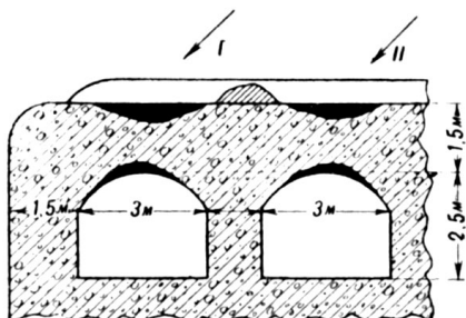
Черт. 17. Попадание 21-см бомб в бетонные своды толщ. 1,5 м.
