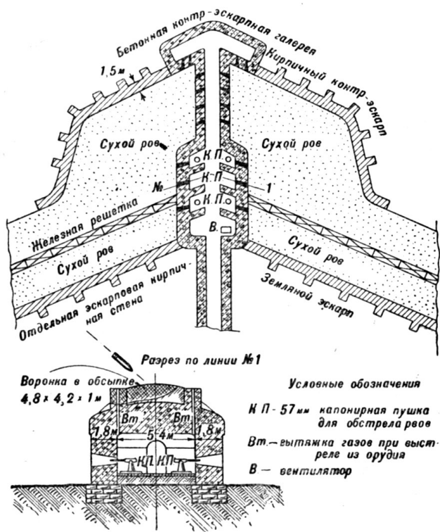
Черт. 8. Капонира № 5 Центрального форта
