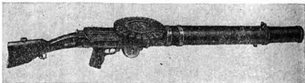
Английский ручной пулемёт «Льюис» образца 1915.
