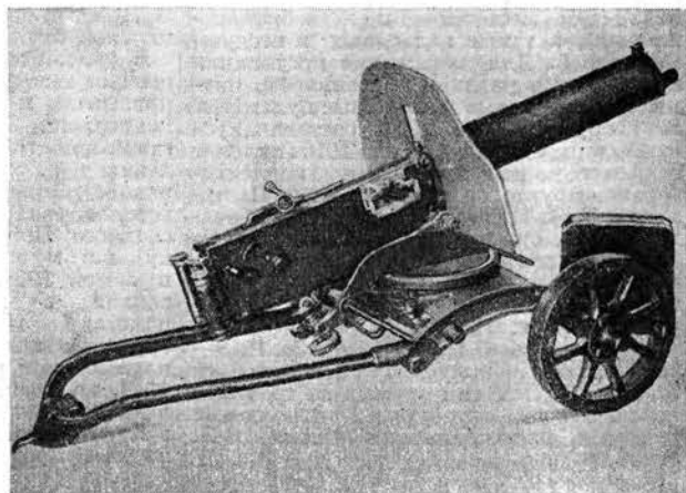
Станковый пулемёт Максима образца 1910.
