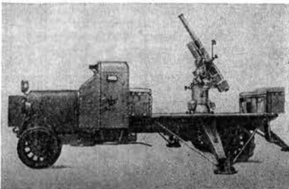
3-дюймовая зенитная пушка в боевом положении на автомобиле.
