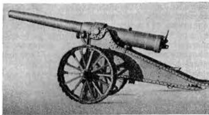
6-дюймовая осадная пушка образца 1904.
