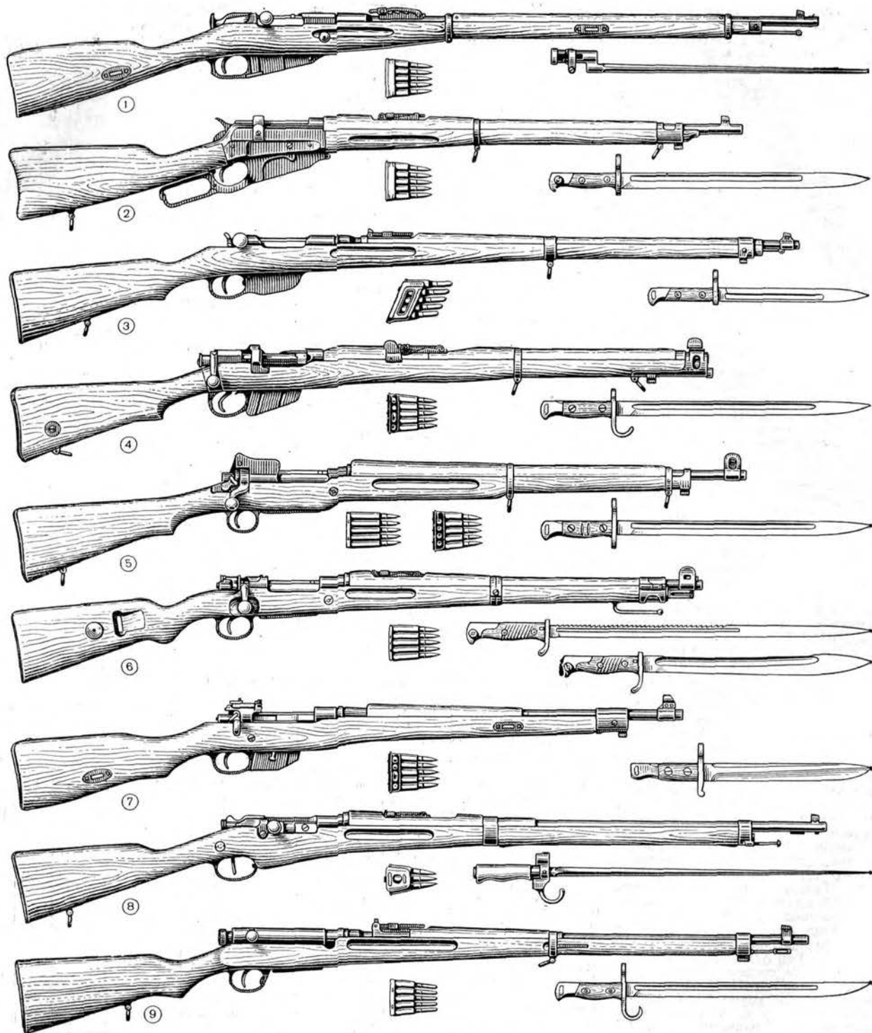
Винтовки: 1—3-линейная (7,62-мм) пехотная системы Мосина образца 1891 (Россия). 2—3-линейная системы Винчестер образца 1895 (США). 3—8-мм системы Манлихер образца 1895 (Австро-Венгрия). 4—7,71-мм Ли-Энфилд образца 1903 (Великобритания). 5—Винтовка Энфилд — Маузер. 6—7,92-мм карабин системы Маузер образца 1898/1908 (Германия). 7—7,71-мм карабин Росс образца 1910 (Канада). 8—8-мм системы Лебель образца 1907/15 (Франция). 9—6,5-мм системы Арисака образца 1905 (Япония).
