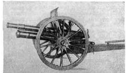
3-дюймовая полевая скорострельная пушка образца 1902.
