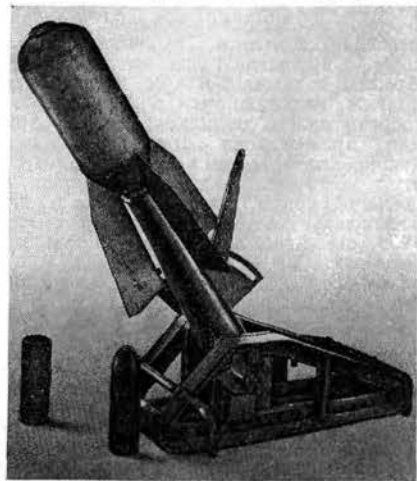
58-мм миномёт Е. А. Лихонина.
