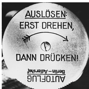
Замок застежки немецкого парашюта
