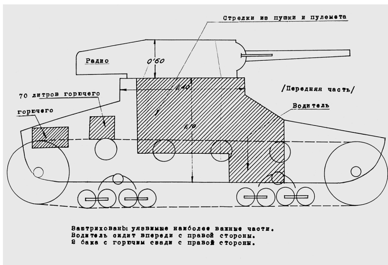
в) Схема танка Т-26
