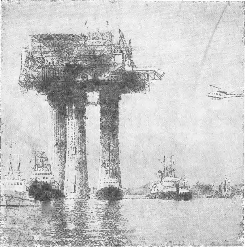
Морская нефтебуровая платформа. Перевозка
