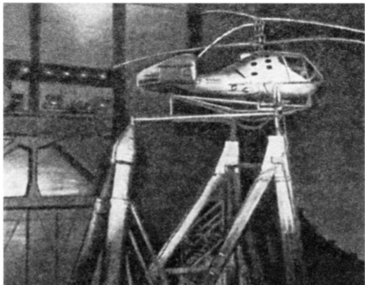
Вертолет Ка-15 испытывается в аэродинамической трубе ЦАГИ. 1953 год.
