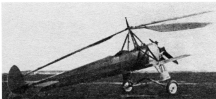
Первый советский винтокрылый аппарат, построенный под руководством Камова – КАСКР-1. Центральный аэродром, 1929 год.
