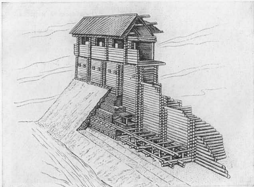
Крепостная стена Белгорода. Конец X в. Реконструкция.
