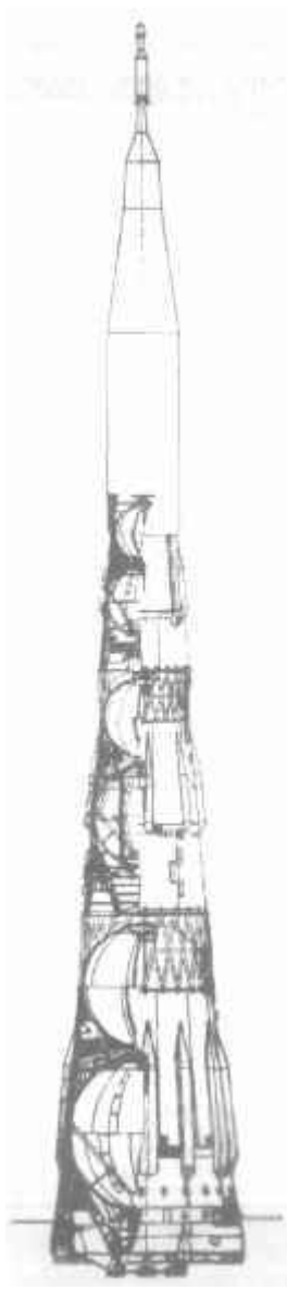
Ракетно-космический комплекс Н1-ЛЗ создавался по Лунной пилотируемой программе
